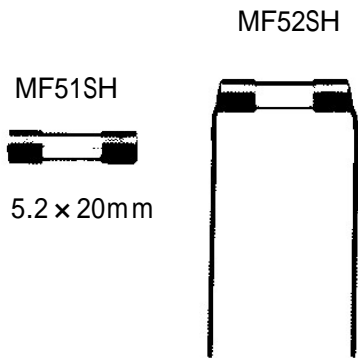
5.2 × 20mm リード線 Lead Wire 0.8 × 35mm: 0.1A ~ 8A 1.0 × 35mm: 10A
